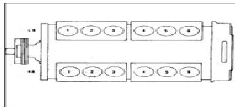
Fig. 7-7. V-1710 Piston position
