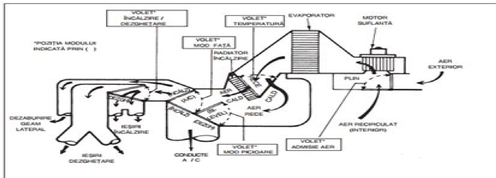
Fig. 3 Schemă curgere aer
