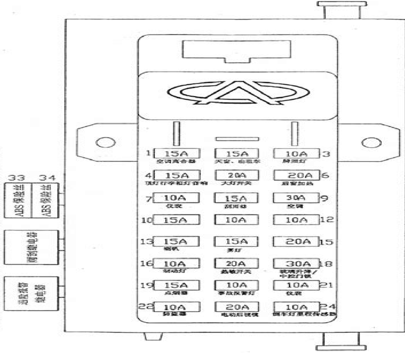
中央电器盒继电器位置图 (室内方向盘下)
