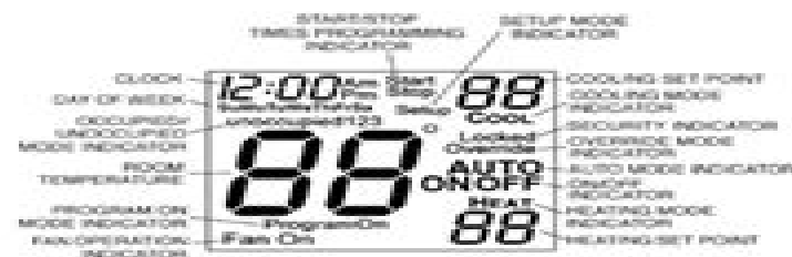
Fig. 1 — Thermostat Display
