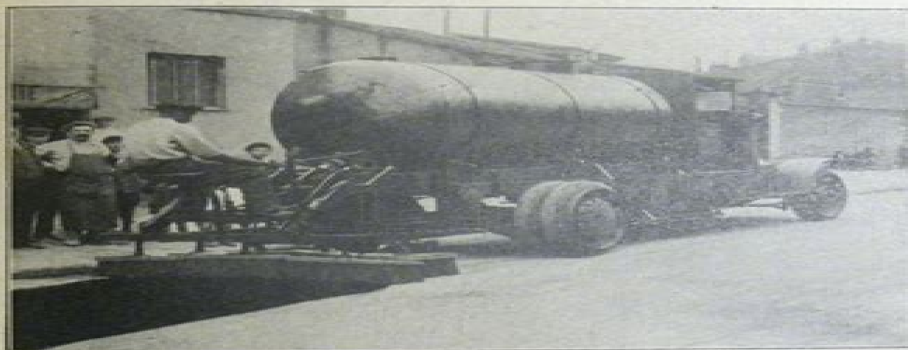
FIG. 23. — Tonne goudronneuse automobile : contenance, 5.000 kgr. (Lassalle).
