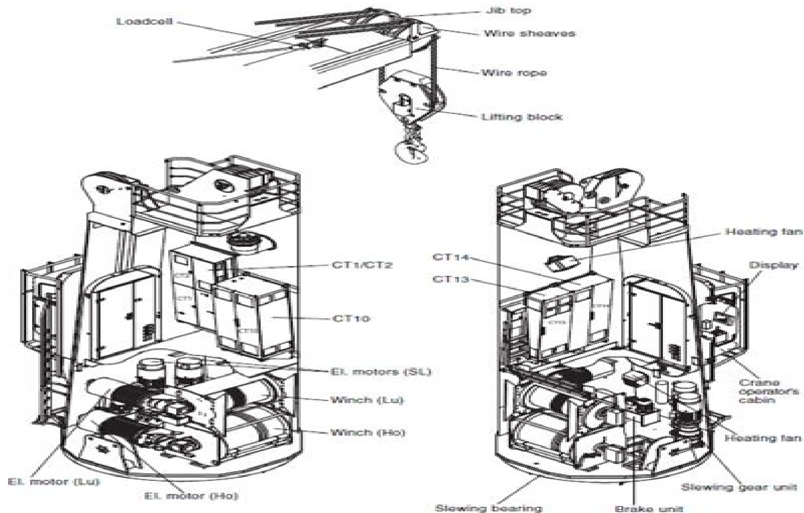
Fig. 1. Crane type GLBE.
